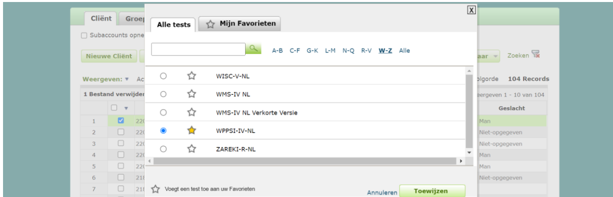
Afbeelding 6 Test toewijzen
